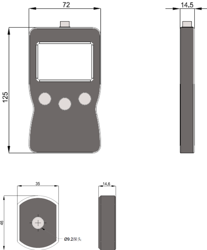
4. FTIU500-275 单波段紫外辐照计外形尺寸：
